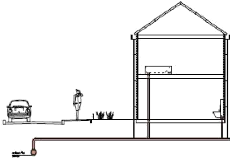
Een gemengd stelsel
